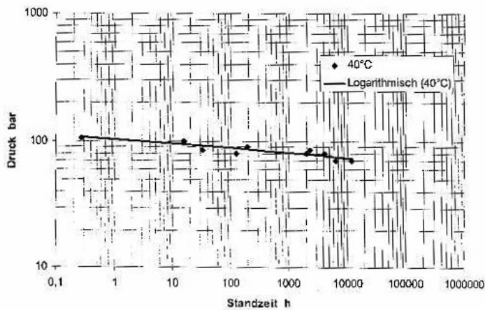
Bild 1: Zeitstand-Innendruckverhalten der Probekörper bei 40 °C
